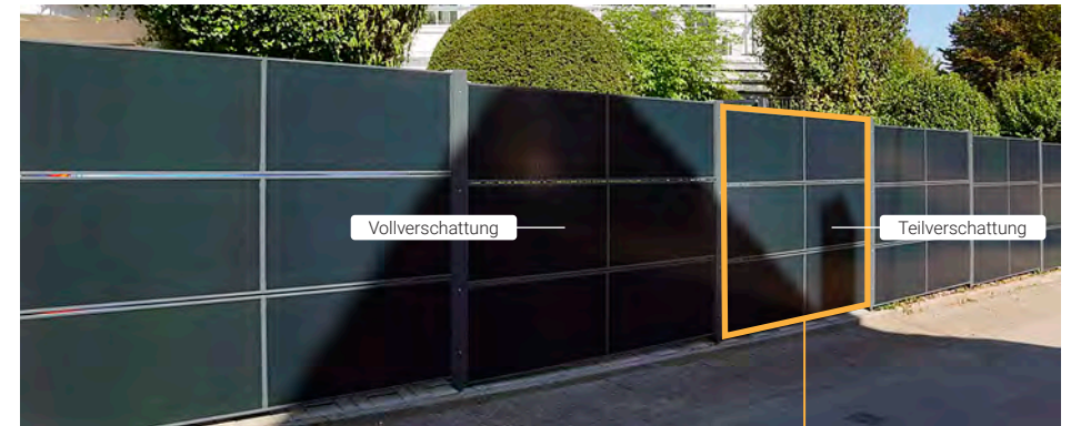
TOP: Beim SolarZaun arbeiten auf einer Fläche von 4,5 m 2 6 parallel verschaltete Photovoltaik-Module.
